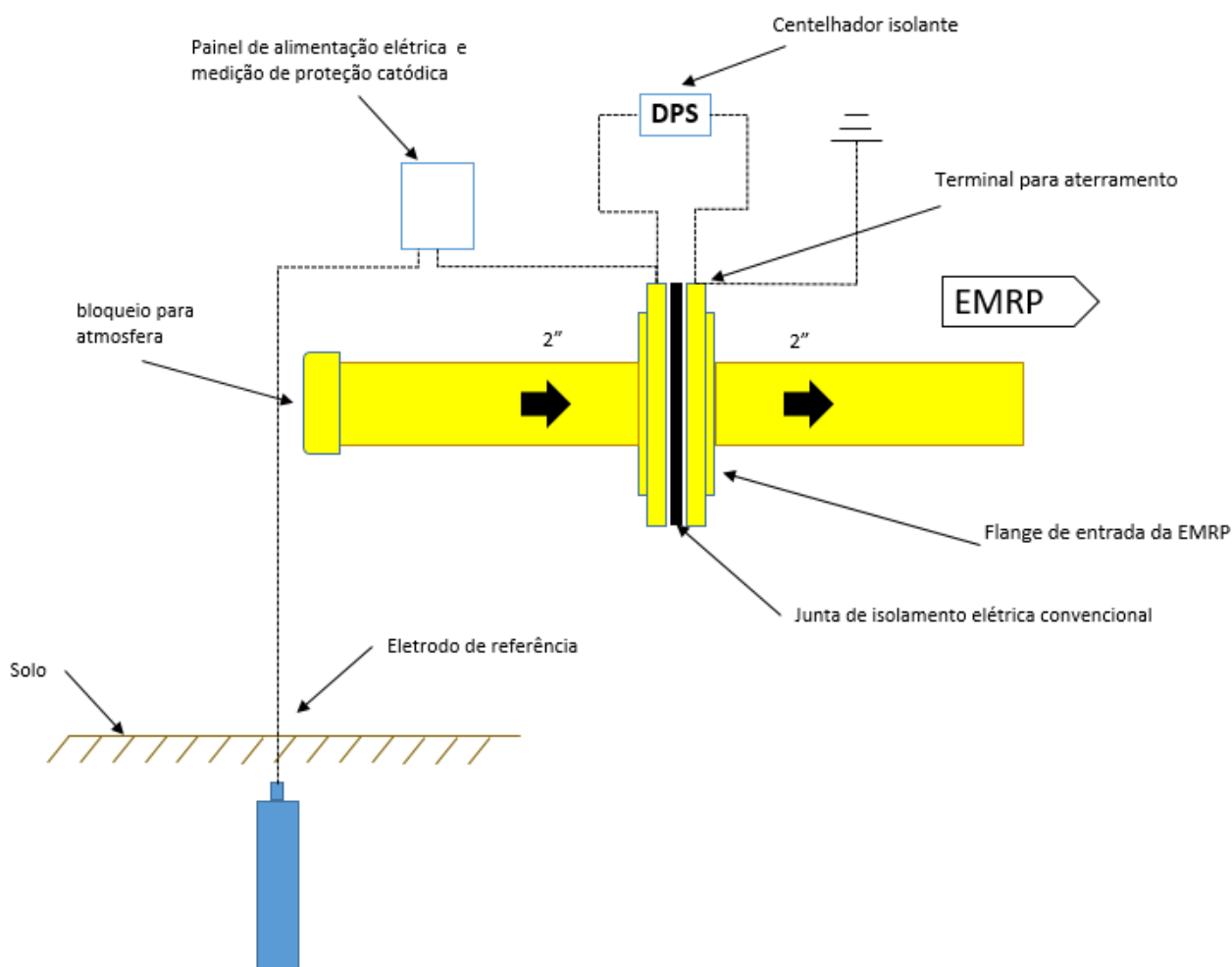
Figura 3 - Medição da proteção catódica.
