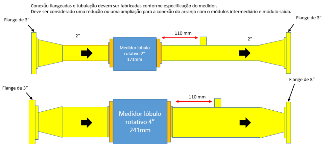
Figura 2- Medição de gás
